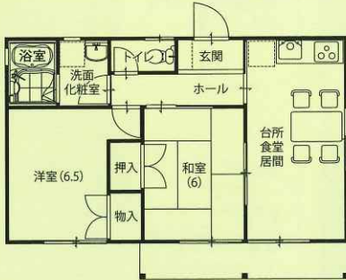
床面積：49.69m 2 (15.03坪)
